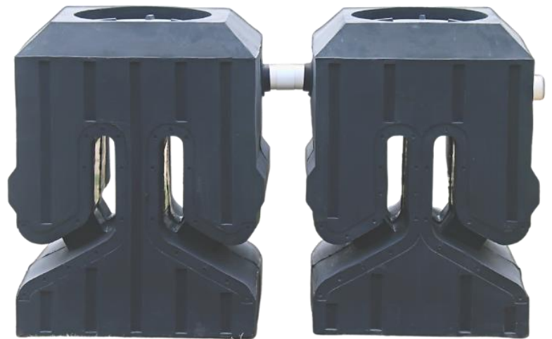
Figura 3. Sistema Individual de Tratamiento de Agua Residual ( SITAR DLD14® ) prefabricado en polietileno.
