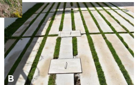
Figura 3. Sistema Individual de Tratamiento de Agua Residual (SITAR DLD14®) construido en panel estructural sin loza (A) en áreas verdes y con loza de seguridad (B) en zona de estacionamiento.
