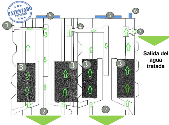
Figura 1. Funcionamiento general del SITAR® DLD 14®.
