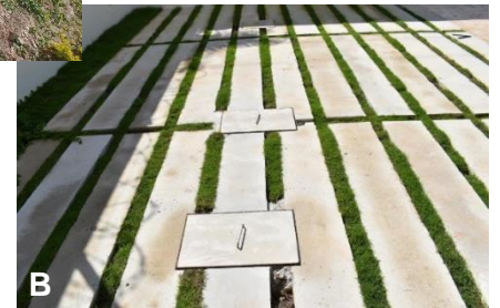
Figura 3. Sistema Individual de Tratamiento de Agua Residual (SITAR DLD14®) construido en panel estructural sin loza (A) en áreas verdes y con loza de seguridad (B) en zona de estacionamiento.
