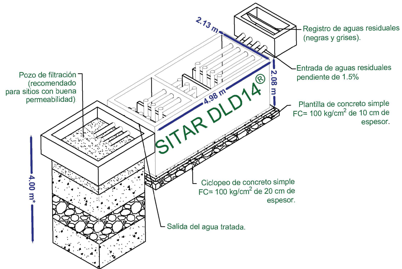
Figura 5. Medidas externas del SITAR DLD14® con Vol.12,525 L/día
