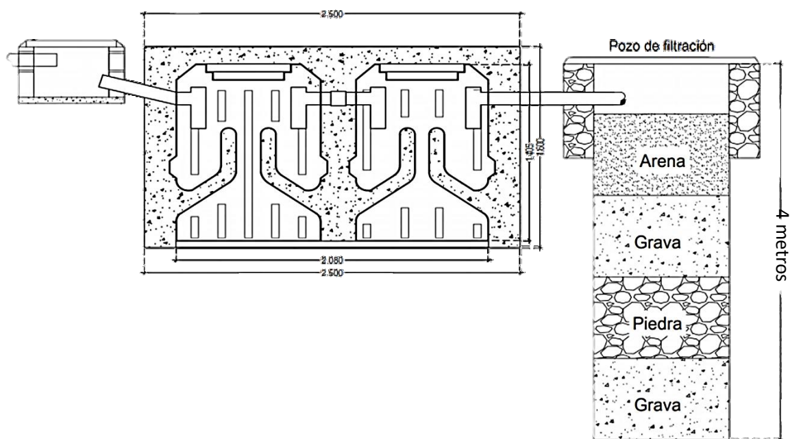
Figura 8. Dimensiones generales y configuración para la instalación adecuada del SITAR DLD14® , corte transversal.
